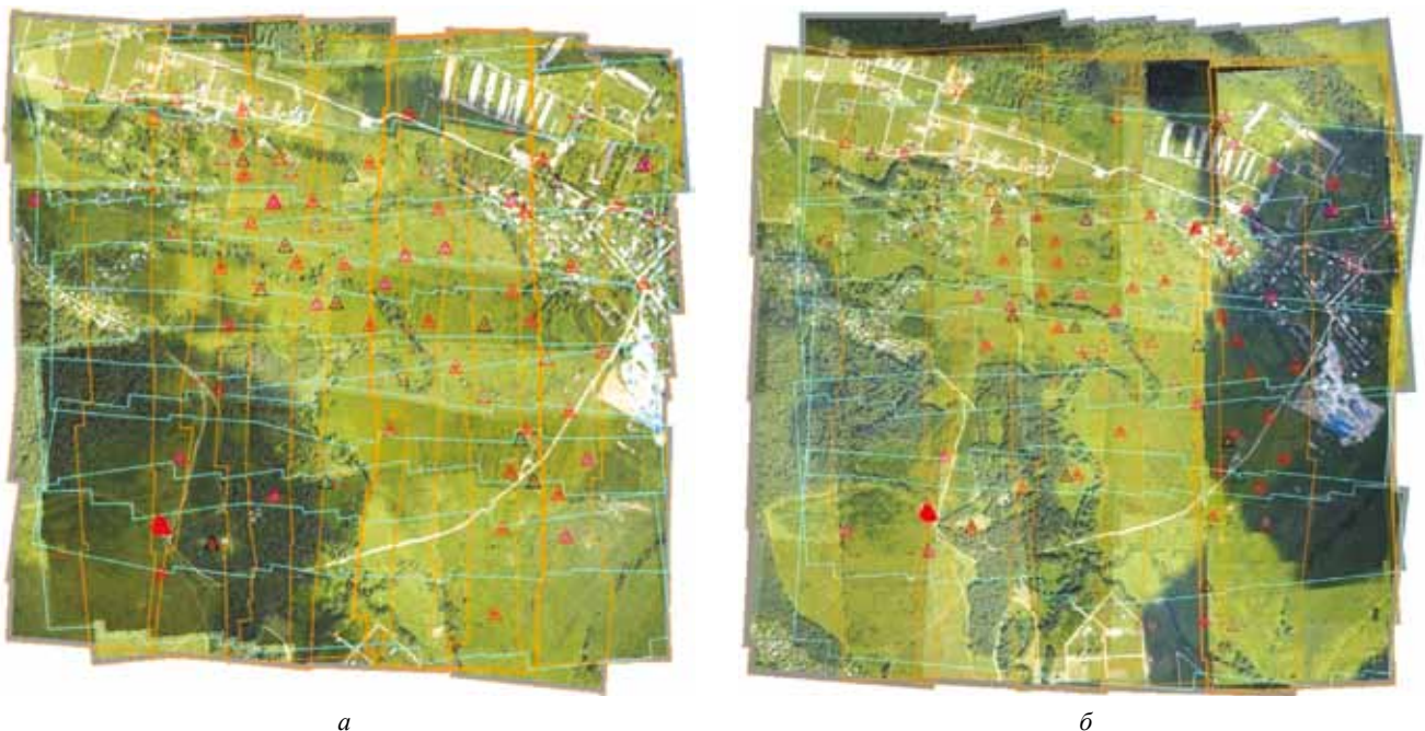
Рис. 3. Схема съемки: а — высота съемки 600 м; б — высота съемки 800 м
